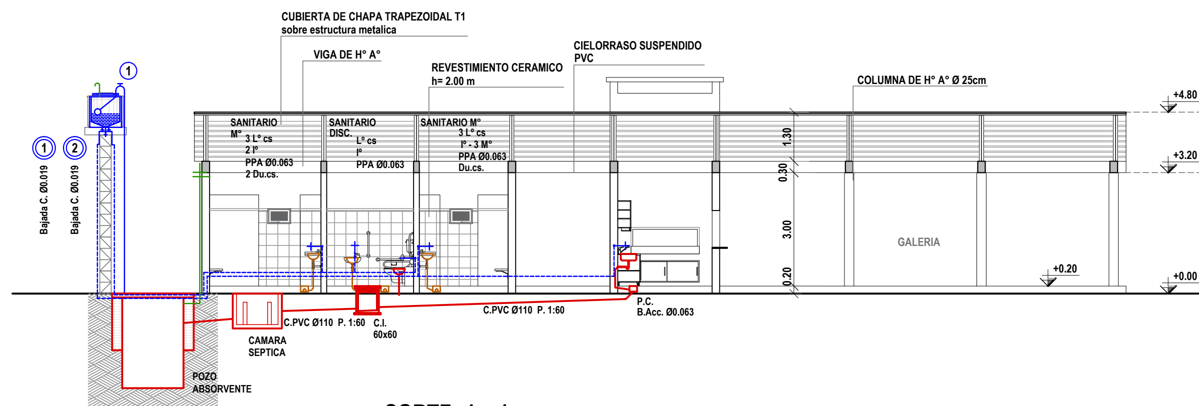
CORTE 1-1
