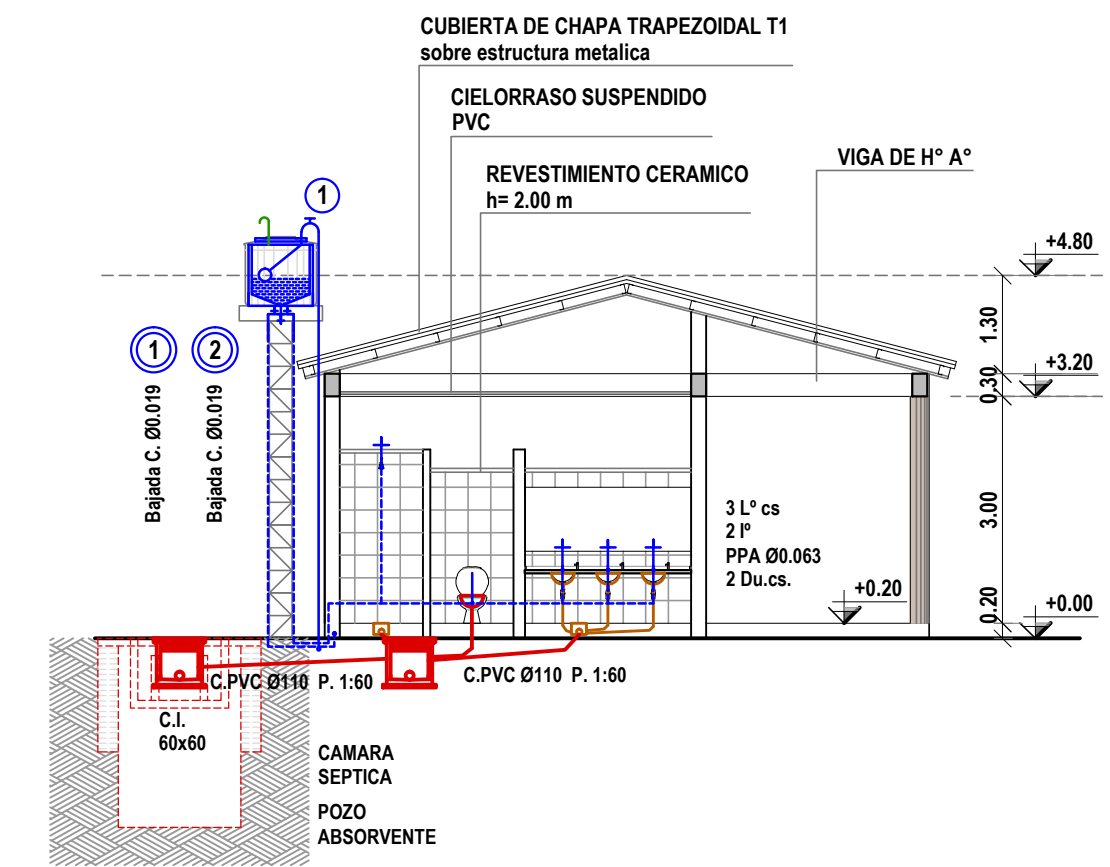
CORTE 2-2
